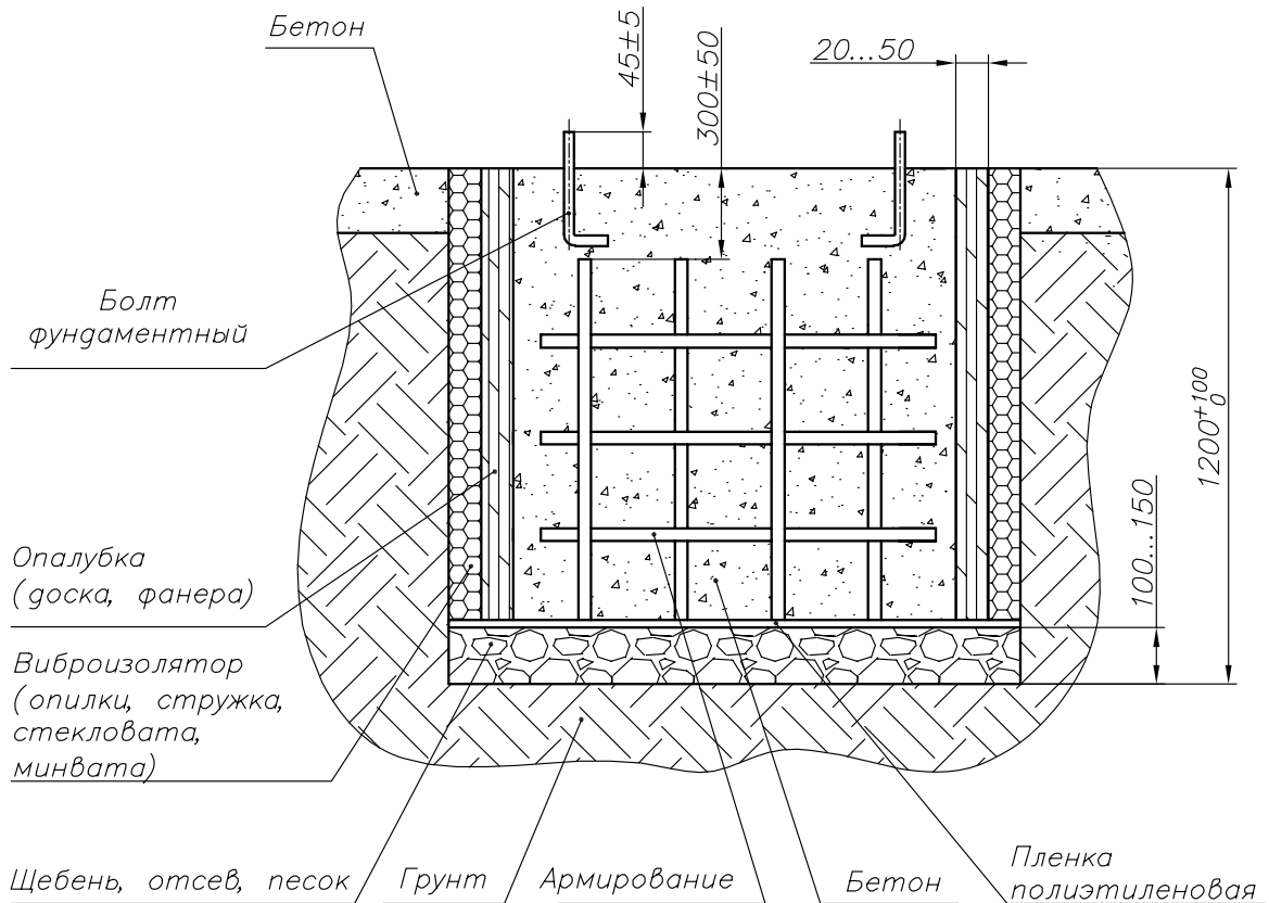
Рис. 18. Сечение фундамента по АА.
